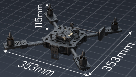
拆卸折叠后最大尺寸（不带桨）
