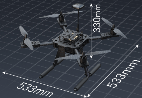
机体展开最大尺寸（带桨）
